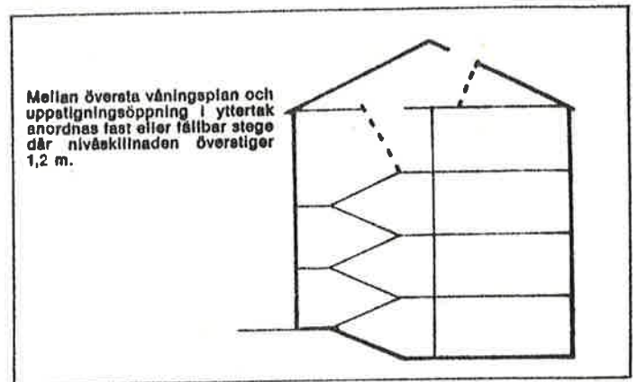
Fig. 5 Exempel på utvändigt uppgång
