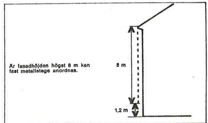
Fig. 8 Uppstigning vid skorstenens nocksida
