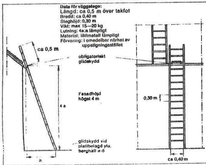
Fig. 6 och 7 Exempel på takanordning från taklucka eller utvändigt steg när taklutningen är mer än 1:4 (14,5°)
