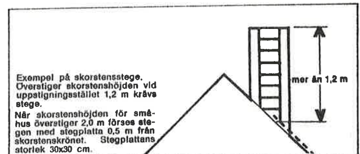
Fig. 10 Uppstigning vid skorstenens gavelnsida
