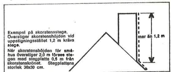
Fig. 10 Uppstigning vid skorstenens gavelnsida
