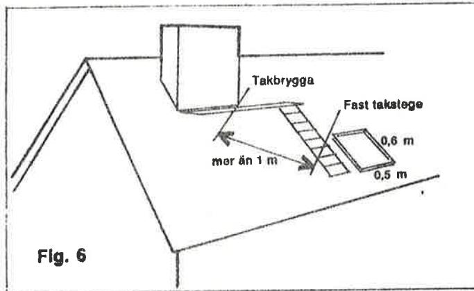
Fig. 6 och 7 Exempel på takanordning från taklucka eller utvändigt steg när taklutningen är mer än 1:4 (14,5°)
