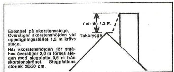
Fig. 9 Uppstigning vid skorstenens takfotsida
